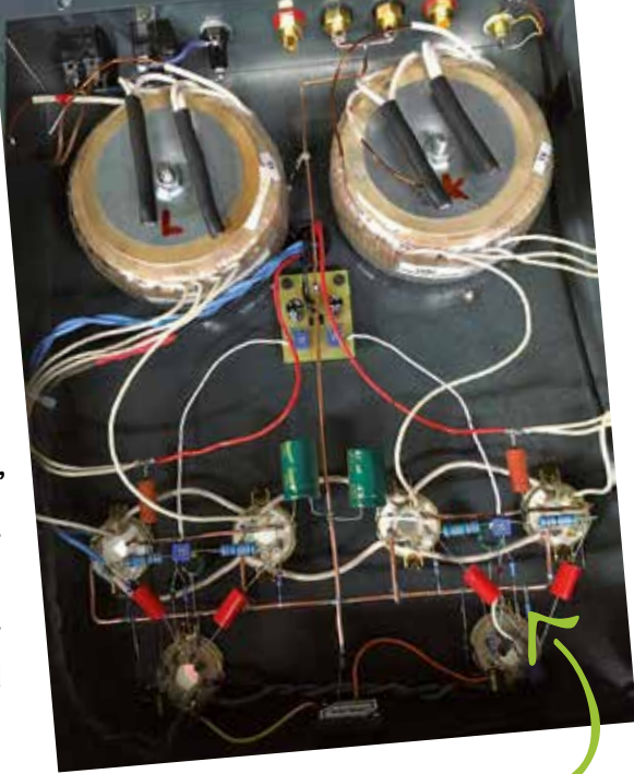
Lampu pastiprinātājs ar platjoslas skaļruņu akustiku. Diezgan sarežģīti!
